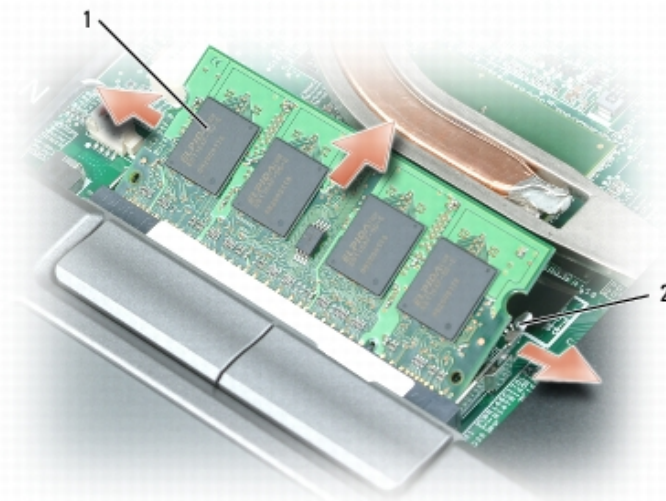
2 תפסי הידוק (2)
