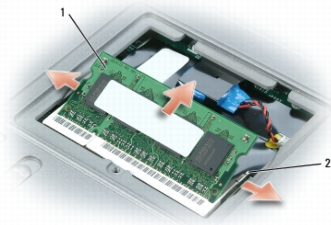
1 מודול זיכרון 2 תפסי הידוק (2)
