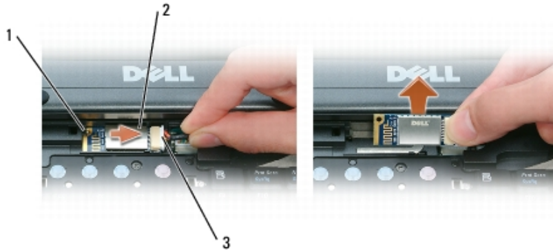
1 לשונית מתכת 2 כרטיס 3 מחבר כבל
